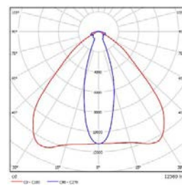
Тип КСС: 90°/30°
