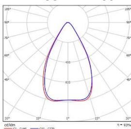
Тип КСС: «Г» - 60°
