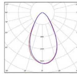
Тип КСС: 60°
