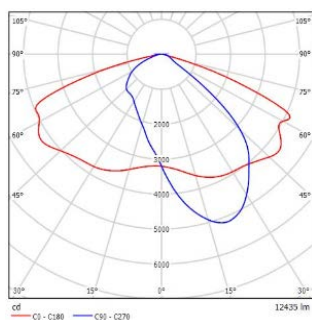
Тип КСС – (ШБ1)
