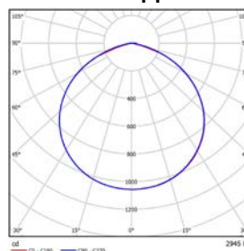
Тип КСС: «Д» - 120°
