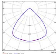
ТИП КСС: «Г-90°»
